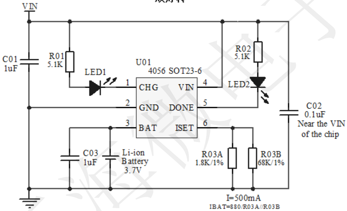
SOT23-6 封装原理图 双灯转
