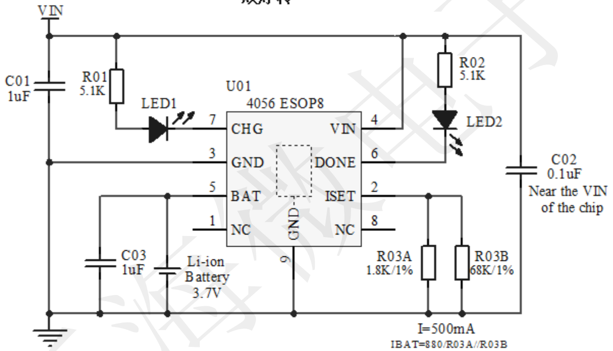
ESOP8 封装原理图 双灯转
