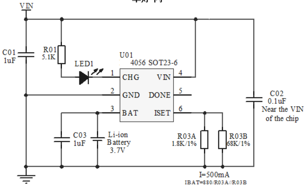
SOT23-6 封装原理图
