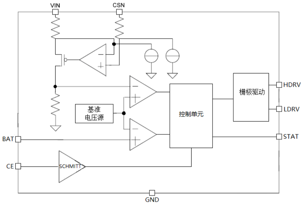
图 3 功能框图
